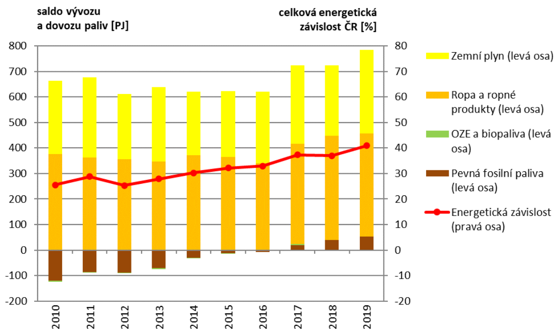
Saldo vývozu a dovozu jednotlivých paliv, dovozní energetická závislost ČR [PJ, %], 2010–2019
