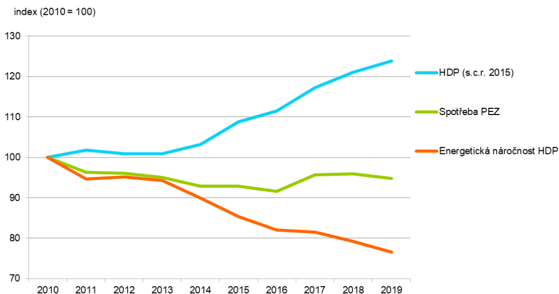
Energetická náročnost HDP v ČR [index, 2010 = 100], 2010–2019
