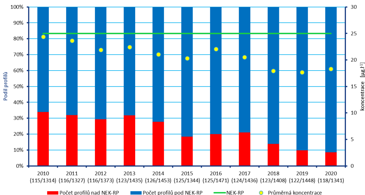
Podíl profilů, kde byl překročen limit NEK-RP pro AOX [%], a průměrná koncentrace [μg.l -1 ], 2010–2020
