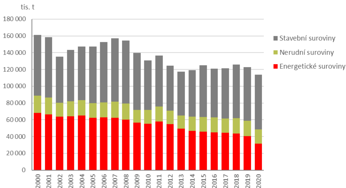
Těžba nerostných surovin v ČR [tis. t], 2000–2020
