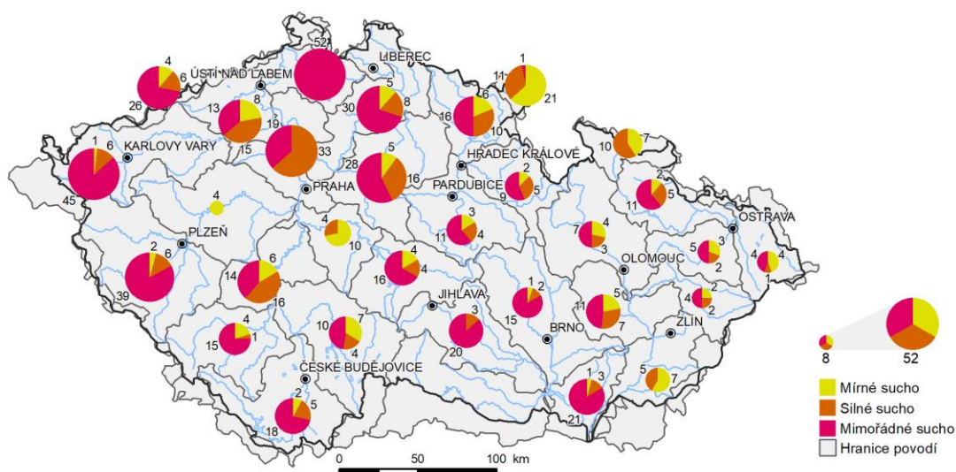
Trvání sucha v pramenech na území ČR [počet týdnů], 2020
