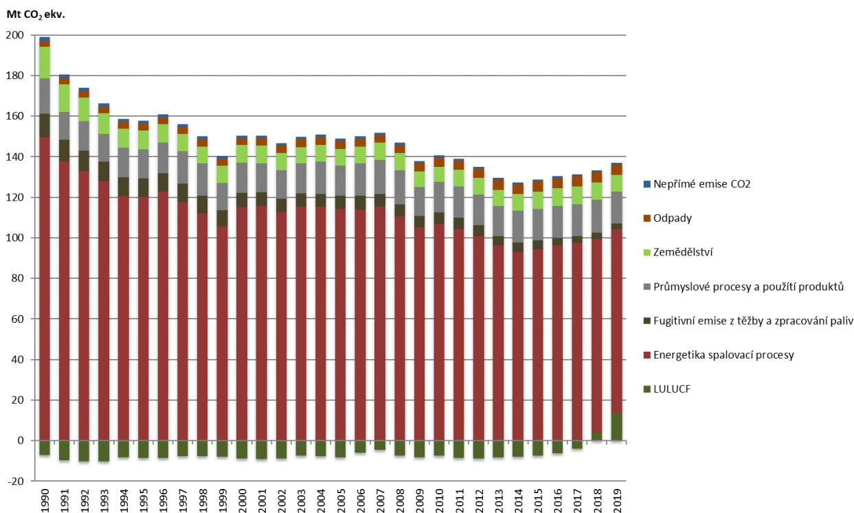
Vývoj agregovaných emisí skleníkových plynů ČR v sektorovém členění [Mt CO 2 ekv.], 1990–2019
