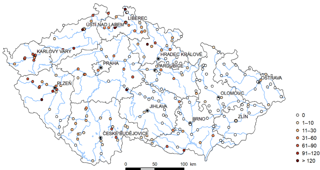
Průtok menší než dlouhodobý 355denní průtok na území ČR za období 1981–2010 [počet dní], 2020
