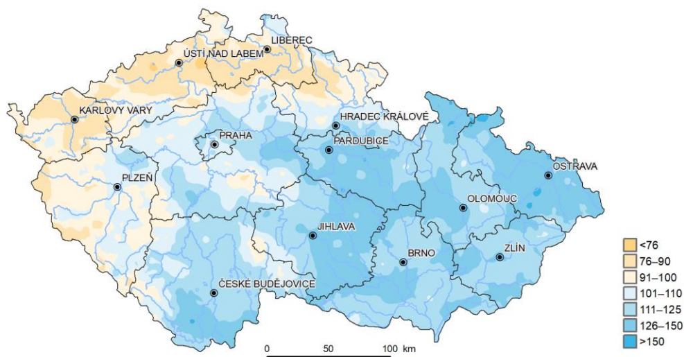
Úhrn srážek v % srážkového normálu 1981–2010 [%], 2020
