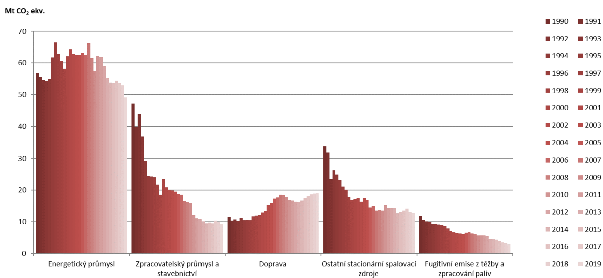
Vývoj emisí z jednotlivých kategorií energetických procesů (CRF kategorie 1) [Mt CO 2 ekv.], 1990–2019
