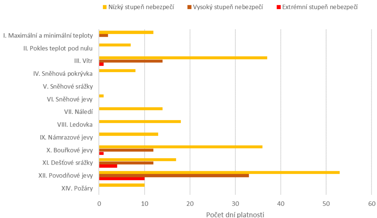
Vydané výstrahy systému SIVS dle skupiny nebezpečného jevu a stupně nebezpečnosti [počet kalendářních dní platnosti výstrahy], 2020
