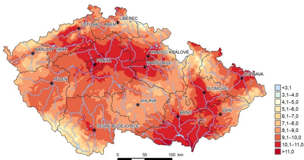
Průměrná roční teplota vzduchu na území ČR [°C], 2020
