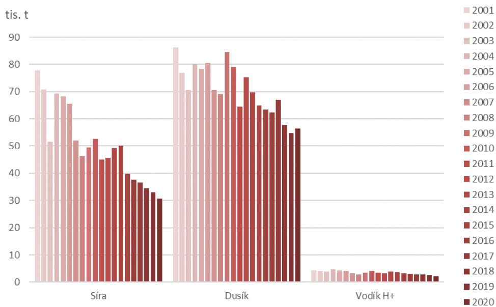
Vývoj celkové atmosférické depozice síry, dusíku a vodíkových iontů v ČR [tis. t], 2001–2020
