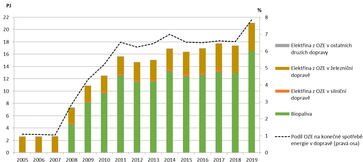
Spotřeba energie z OZE v dopravě v ČR a podíl OZE na konečné spotřebě energie v dopravě [PJ, %], 2005–2019
