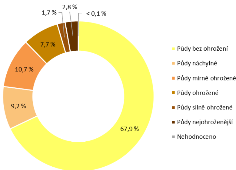
Potenciální ohroženost zemědělské půdy větrnou erozí v ČR [% ZPF], 2020
