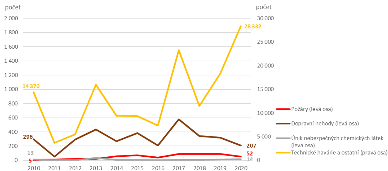
Počet událostí vzniklých v souvislosti se živelními pohromami v ČR, 2010–2020
