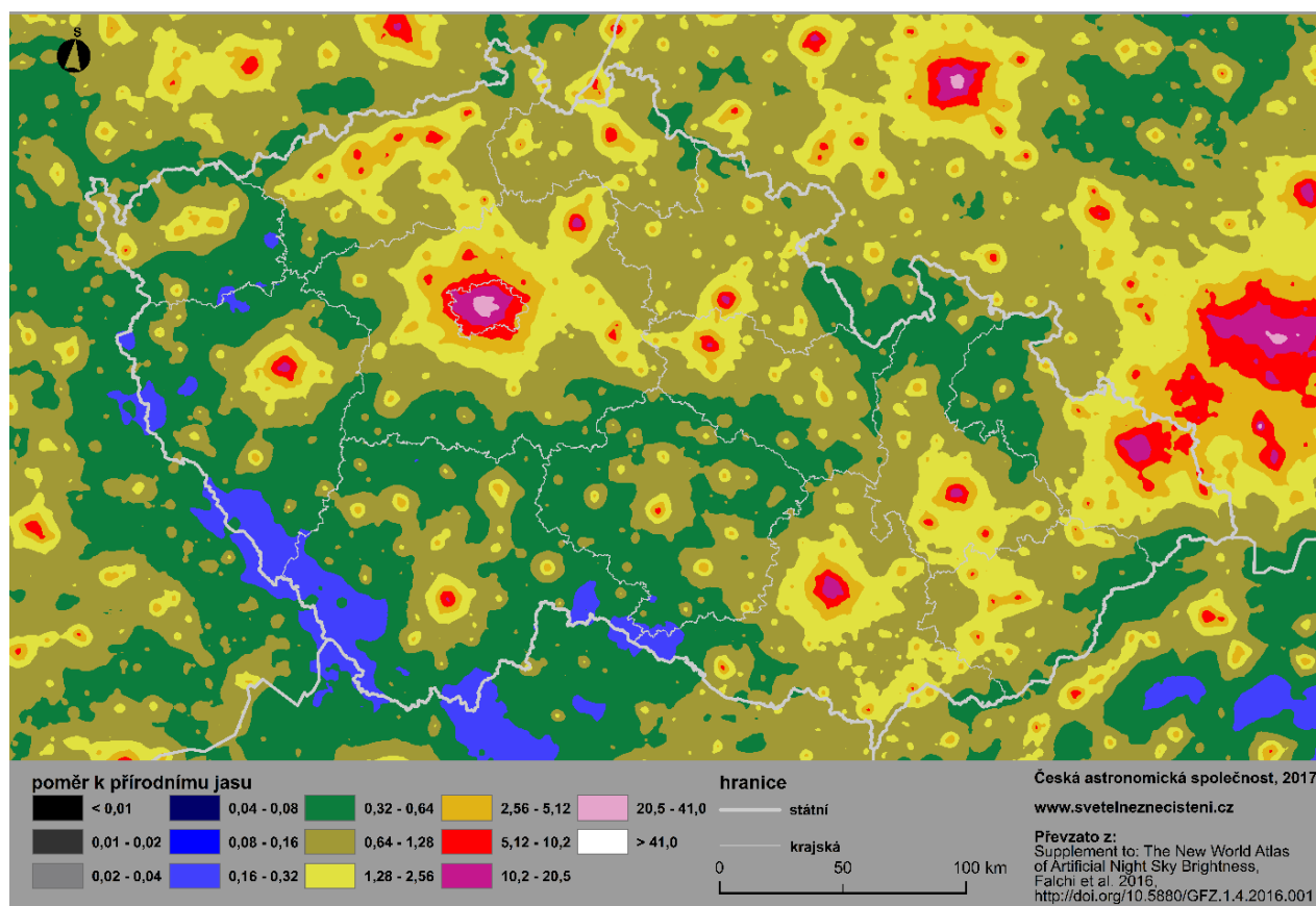
Umělý jas noční oblohy nad ČR, 2016
