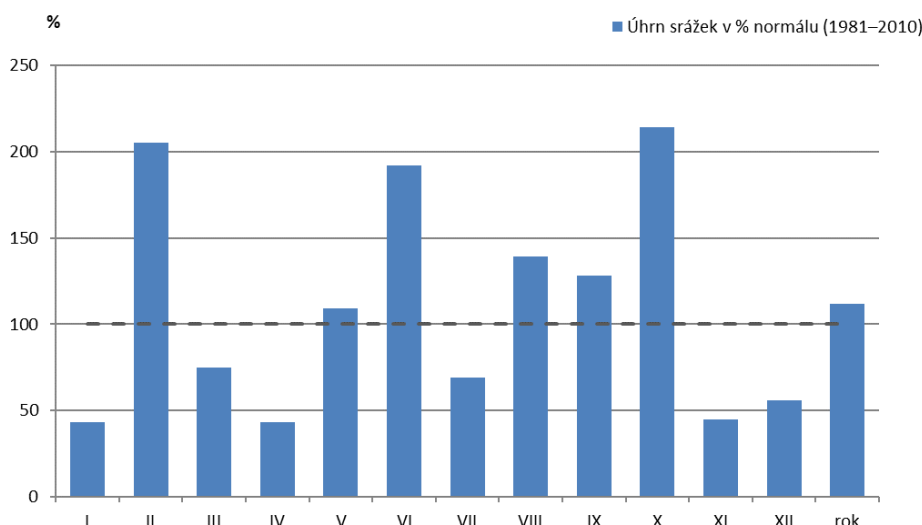
Měsíční úhrn srážek v % normálu 1981–2010 [%], 2020
