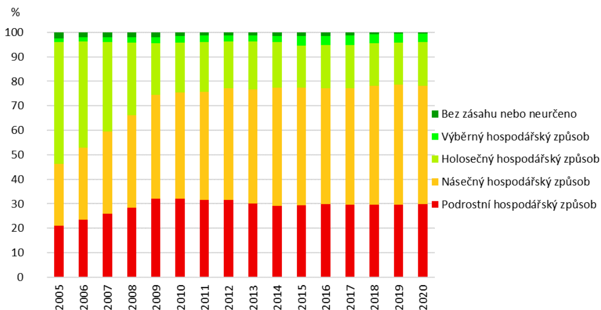
Rozloha lesů ČR rozdělená dle hospodářského způsobu v LHP [%], 2005–2020
