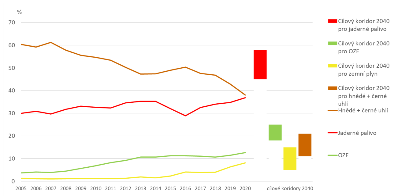
Podíl výroby elektřiny podle druhu paliv v ČR [%], 2005–2020
