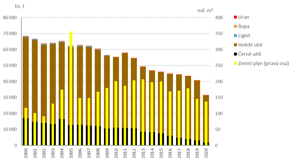
Těžba energetických surovin v ČR [tis. t, mil. m 3 ], 2000–2020
