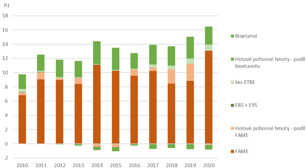
Spotřeba biopaliv v ČR a bilance dovozu a vývozu biopaliv v hotových pohonných hmotách [PJ], 2010–2020
