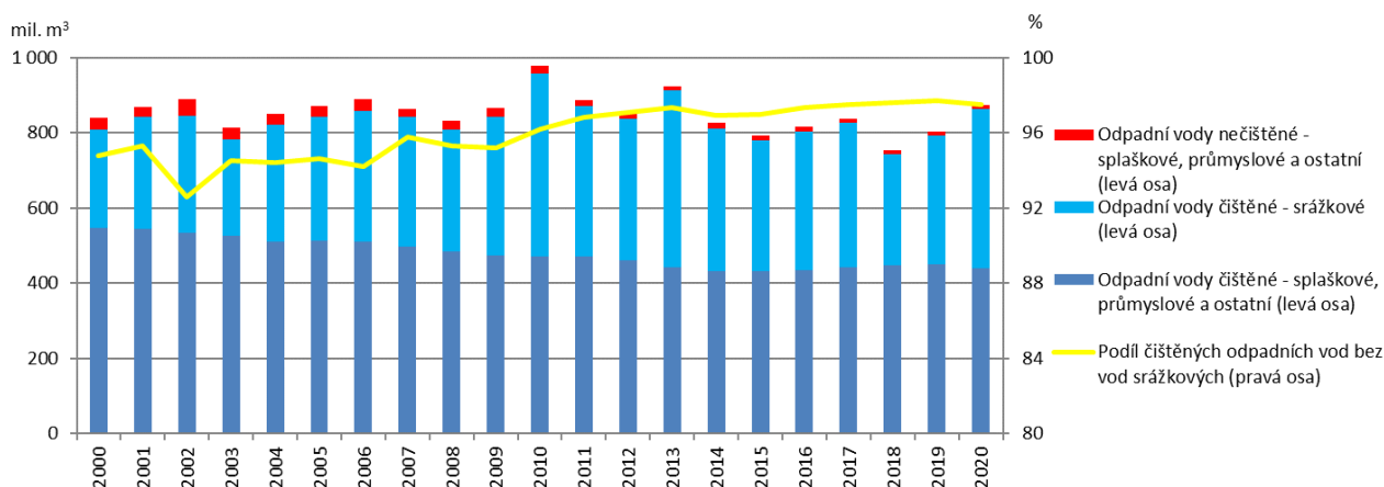
Čištění odpadních vod vypouštěných do kanalizace v ČR [mil. m 3 , %], 2000–2020
